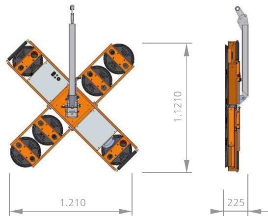
Basisgerät mit Erweiterung 1 und Anschlussflanschen Basic device with enlargement 1 and lateral coupling flanges
