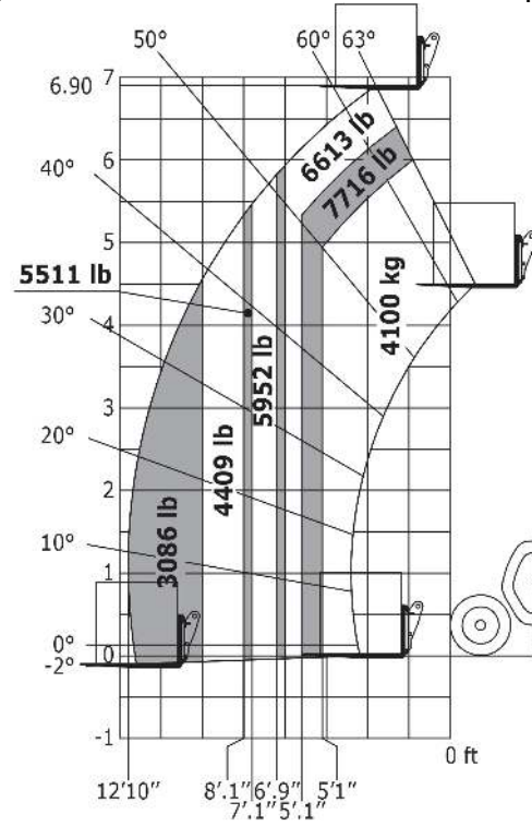
Rough terrain load chart (EN 1459 B) Imperial
